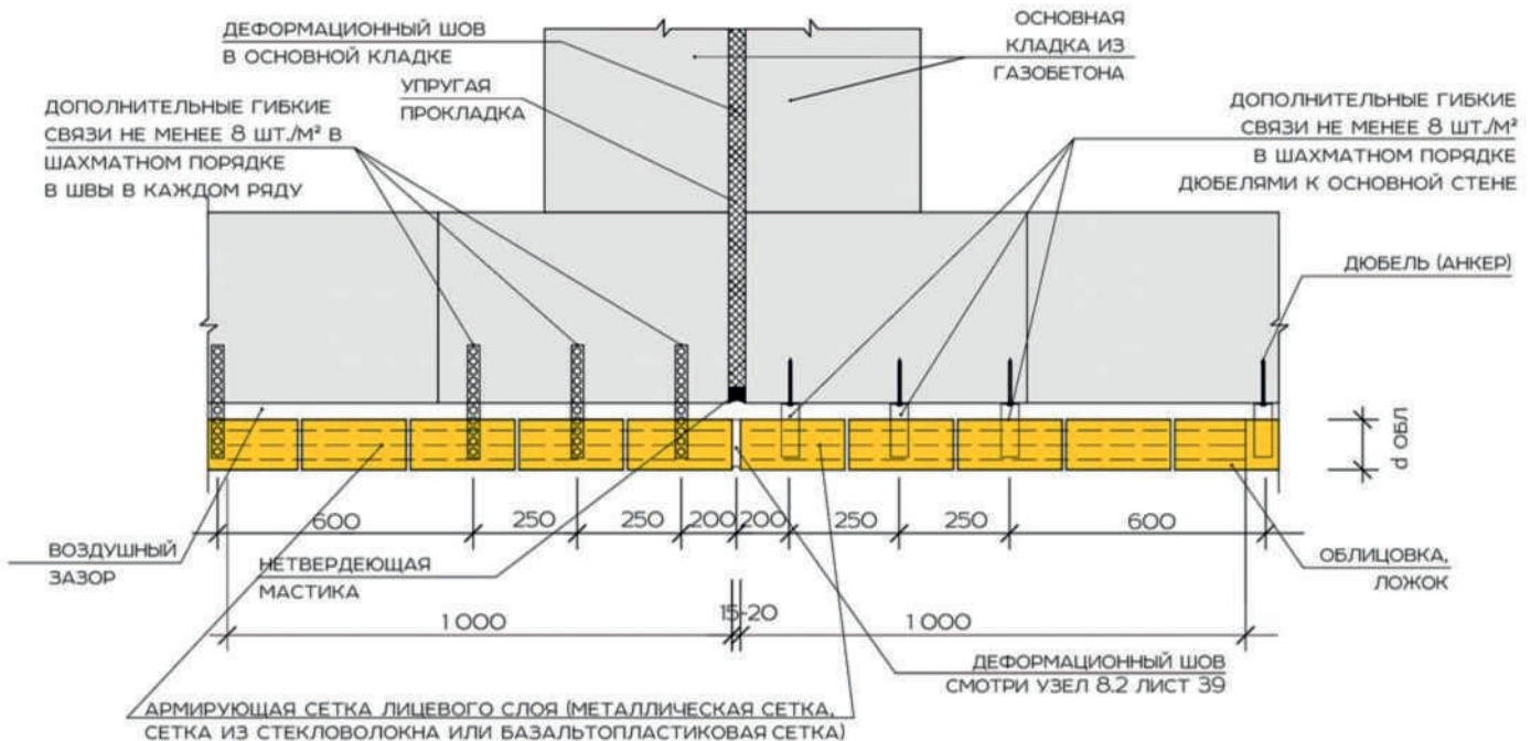
Узел 9.4 РЕШЕНИЕ ДЛЯ ВОЗВОДИМЫХ ЗДАНИЙ СО СТЕНАМИ ИЗ ГАЗОБЕТОНА
