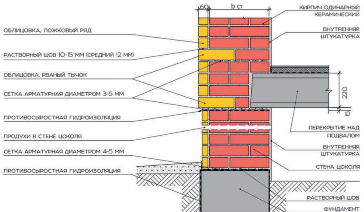
Узел 1.11 ОпираНИЕ КЛАДКИ НА КИРПИЧНЫЙ ЦОКОЛЬ В ЗДАНИЯХ С ВЕНТИЛИРУЕМЫМ ТЕХПОДПОЛЬЕМ
