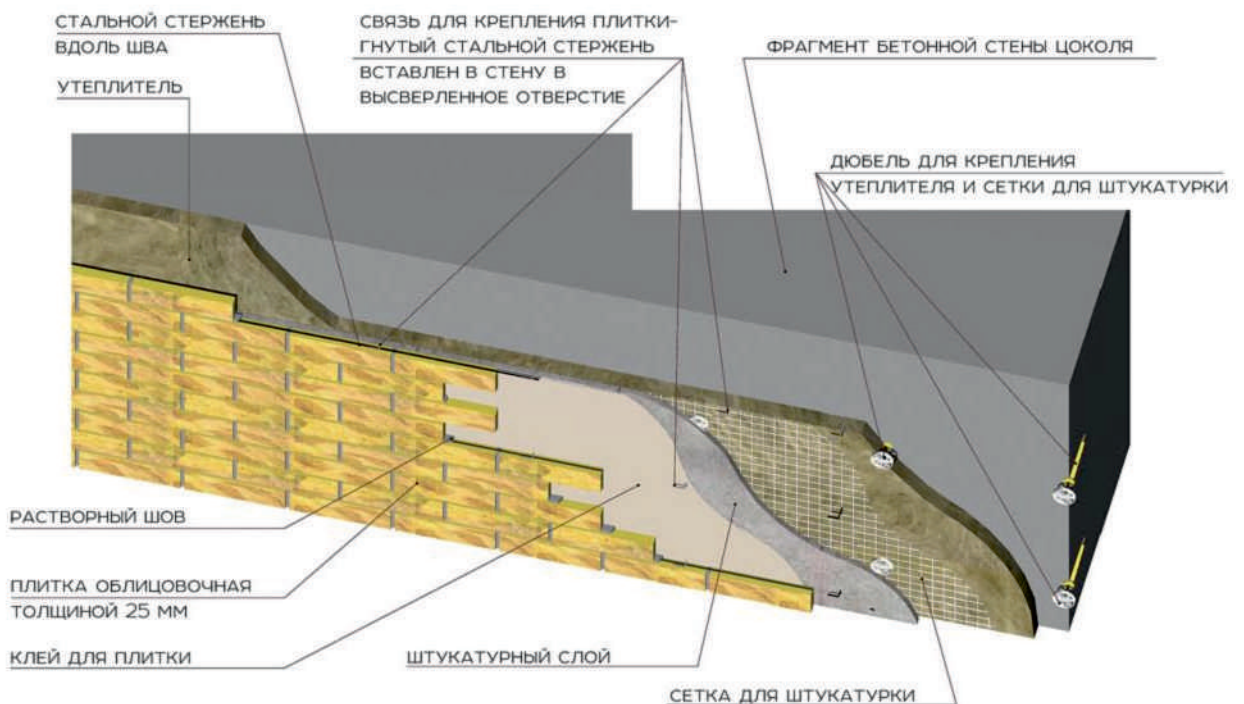
Узел 6.2 Устройство облицовки цокольной стены из бетона с утеплителем
