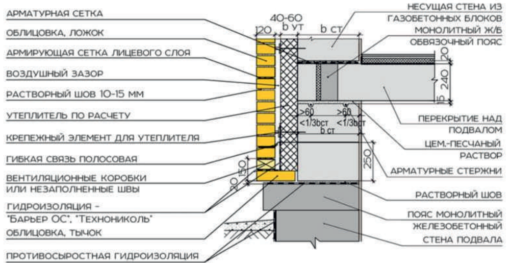
Узел 4.3 ОпираНИЕ КЛАДКИ НА ГАЗОБЕТОННЫЙ ЦОКОЛЬ В ЗДАНИЯХ С ВЕНТИЛИРУЕМЫМ ТЕХПОДПОЛЬЕМ
