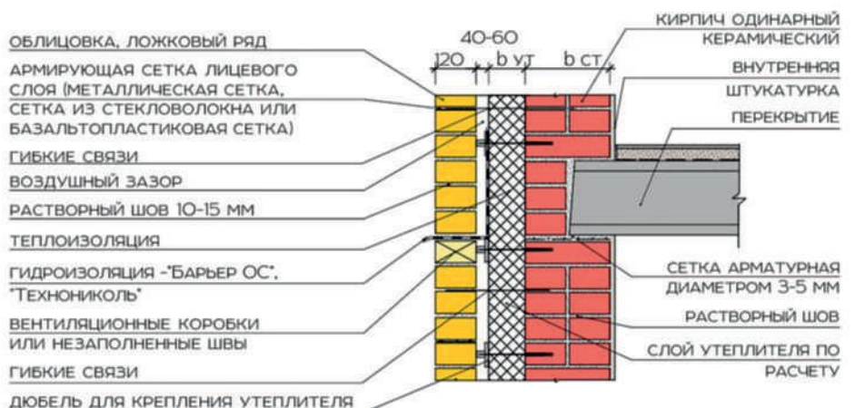
Узел 3.4 ОпираНИЕ межэтажных перекрытий на кирпичную кладку с облицовкой
