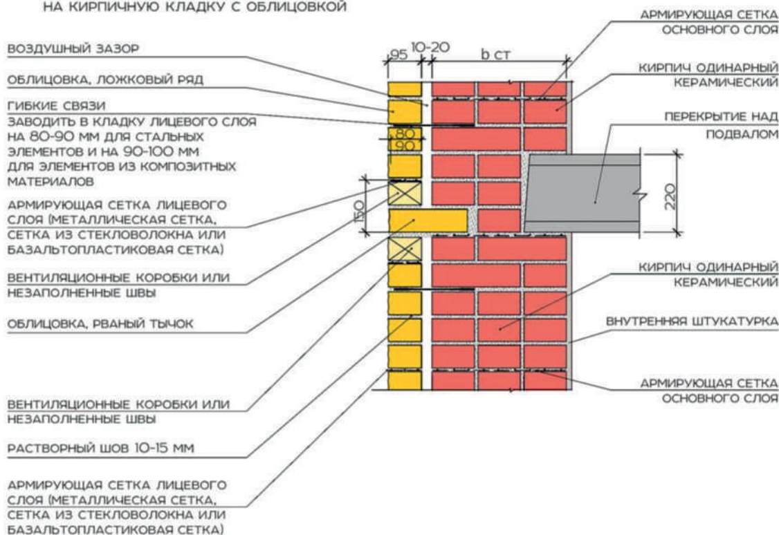
Узел 1.20 Опирание межэтажных перекрытий на кирпичную кладку с облицовкой
