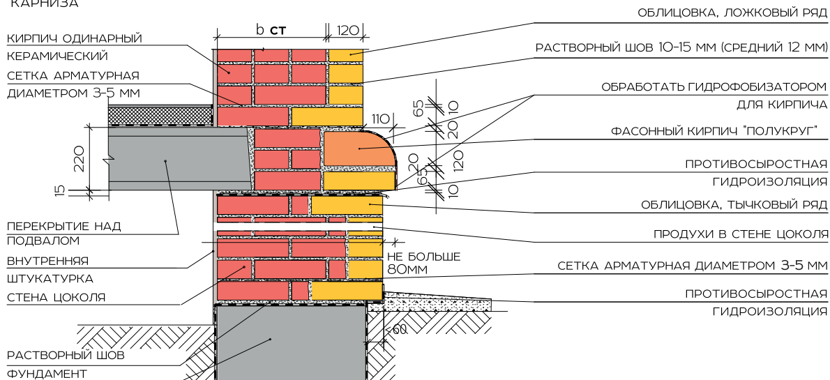
Узел 10.2 Устройство междуэтажного карниза, сечение
