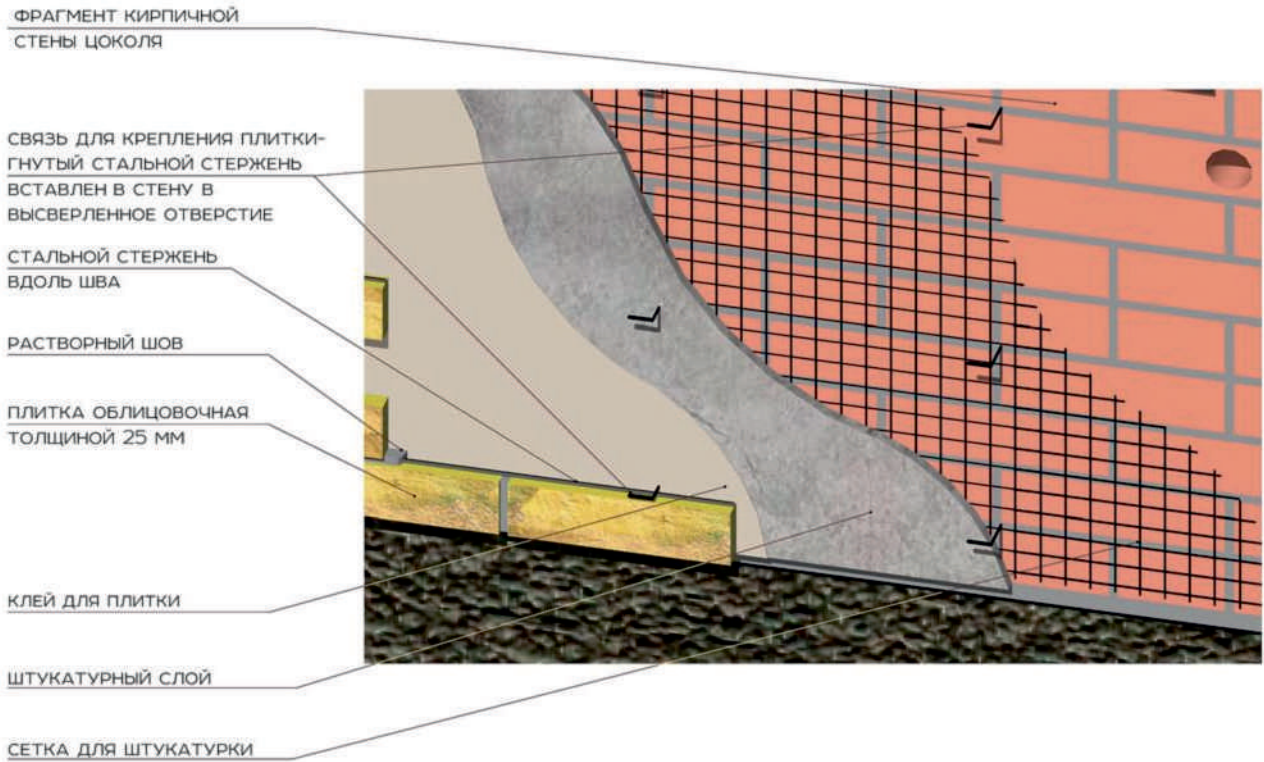
Узел 6.1 Устройство облицовки цокольной СТЕНЫ ИЗ КИРПИЧА
