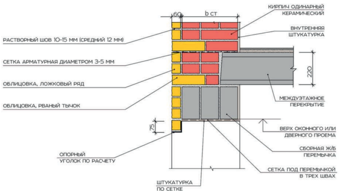
Узел 1.12 ОпиРАНИЕ МЕЖЭТАЖНЫХ ПЕРЕКРЫТИЙ НА ОБЛИЦОВАННУЮ КИРПИЧНУЮ СТЕНУ С ПРОЕМОМ
