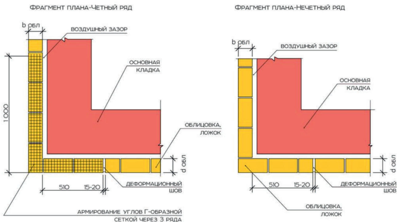
Узел 8.2 Деформационный шов в лицевом слое
